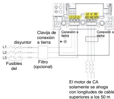
Red eléctrica en los terminales del motor
